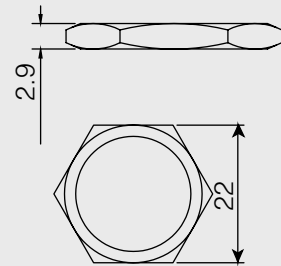
Hex Nut
